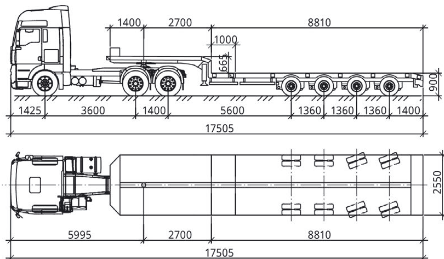
Автопоезд в компактном состоянии
