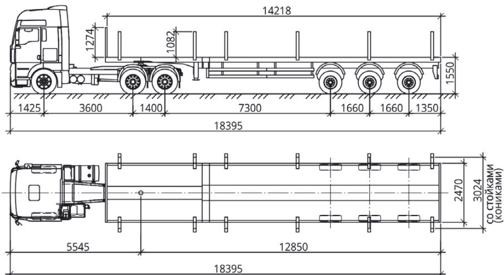
Автопоезд в раздвинутом состоянии
