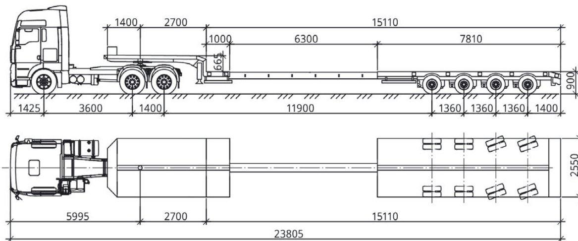
Автопоезд в раздвинутом состоянии
