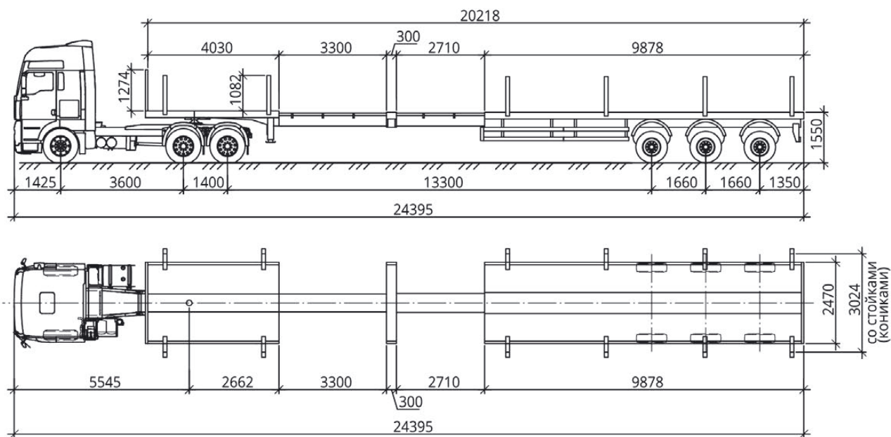
Автопоезд в раздвинутом состоянии
